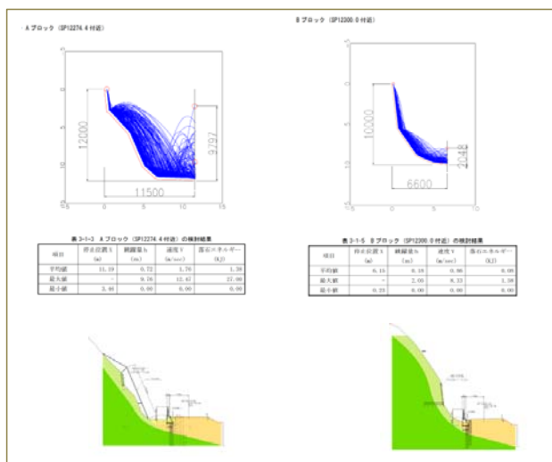
シュミレーション解析と設計断面
